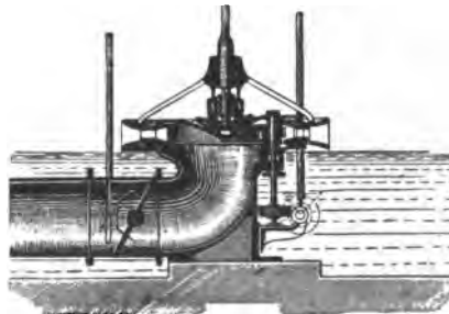
Fig. 52. Girard-Turbine der Maschinenfabrik Geislingen.
